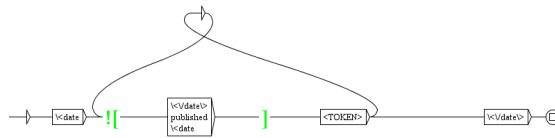
FIGURE 12.24 – Un graphe pour le décompte des balises date dans le fichier standOff, sauf en cas de présence du mot published
