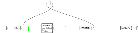
FIGURE 12.26 – Un graphe pour le décompte des balises date dans le fichier standOff, sauf en cas de présence du mot published
